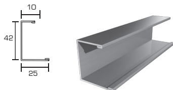
PROFILO A "C" 25X42X10 L=4000 mm
