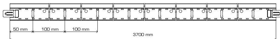
Main T (Rak T-profil) 3700 mm
