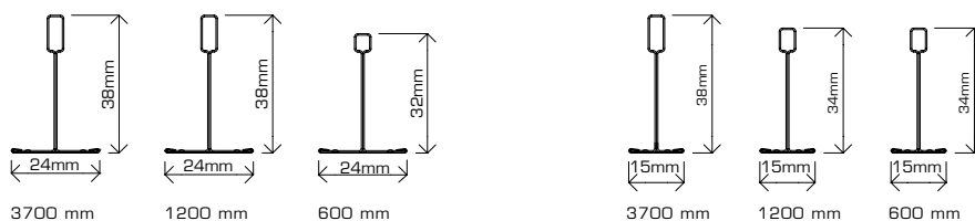
Main T (Rak T-profil) 3700 mm
