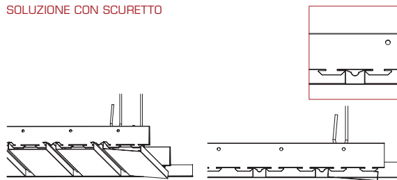
SOLUZIONE CON SCURETTO
